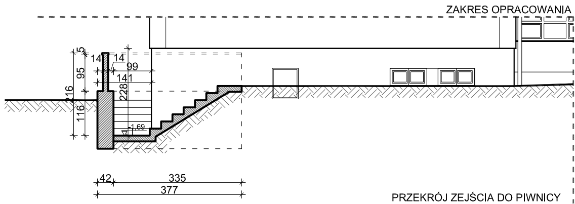
PRZEKRÓJ ZEJŚCIA DO PIWNICY
